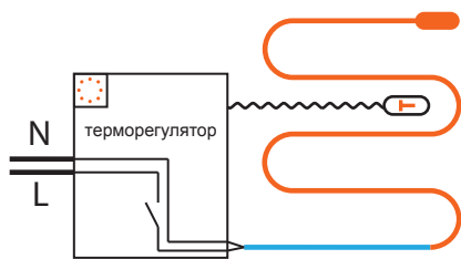
Схема электрического подключения через терморегулятор
