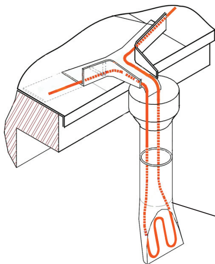
Схема монтажа на кровле и водостоках
